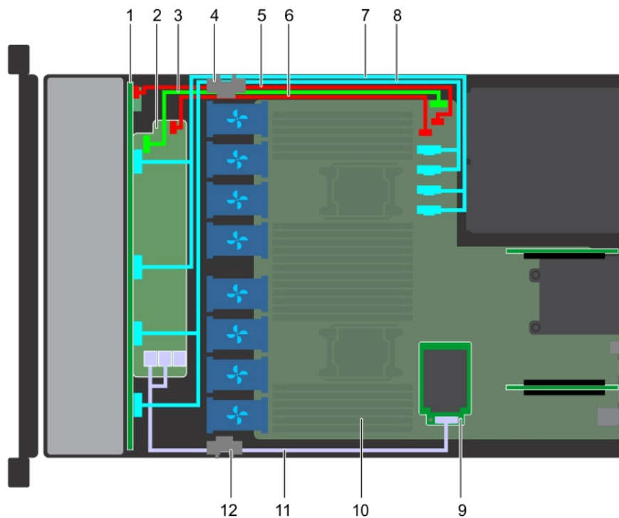
图 62: 电缆布线 - 10 x 2.5 英寸硬盘驱动器背板
