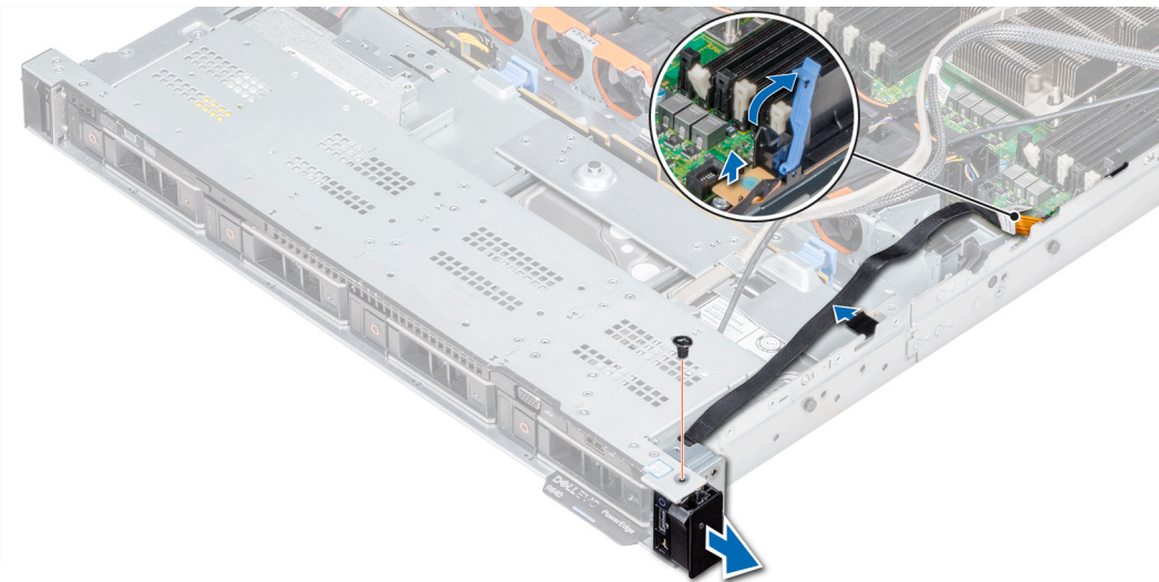
图 80: 卸下右控制面板
