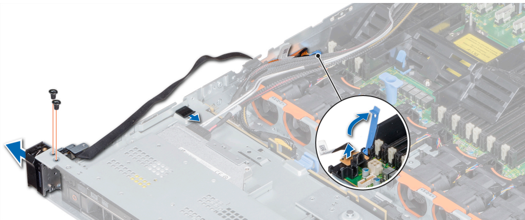
图 76: 卸下左控制面板
