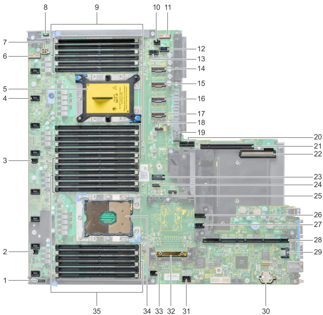
图 83: 系统板跳线和连接器
