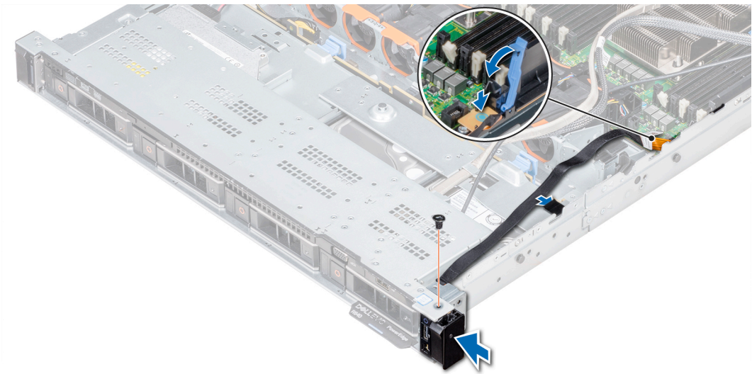
图 81: 安装右控制面板
