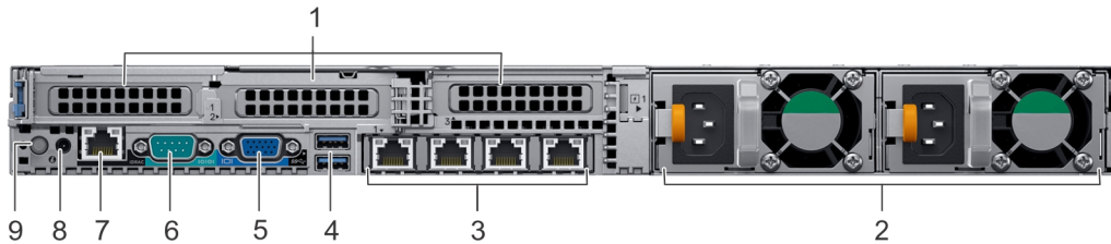
图 7: 具有三个 PCIe 扩展槽的设系统的背面视图
