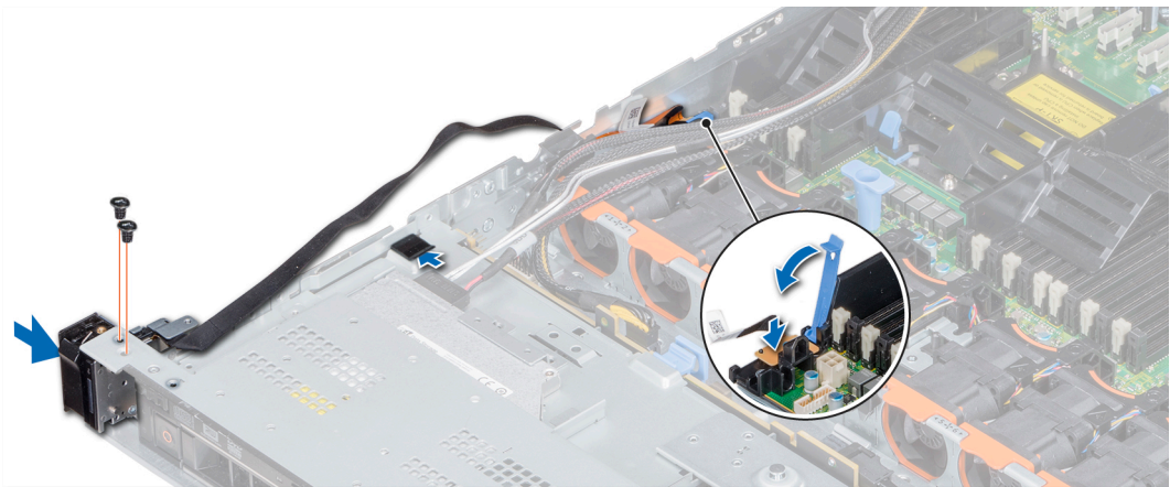
图 77: 安装左控制面板
