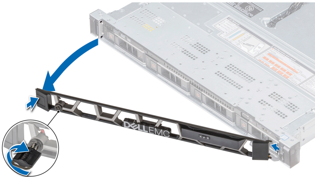
图 14: 卸下带 LCD 面板的可选前挡板
