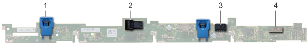
图 60: 4 x 3.5 硬盘驱动器背板
