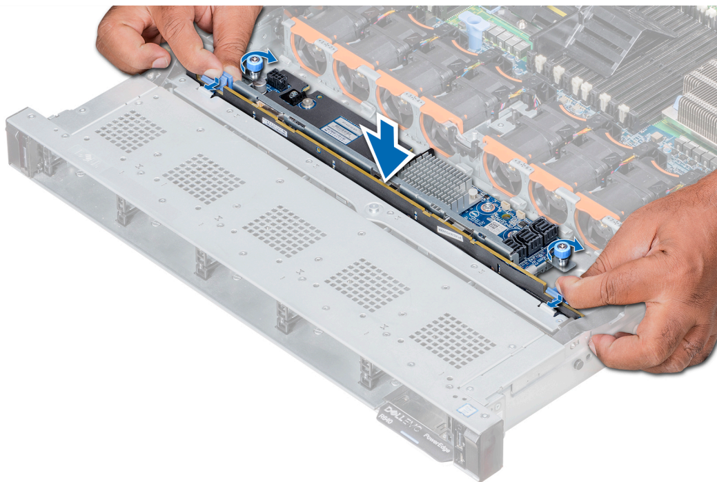
图 61: 安装硬盘驱动器背板
