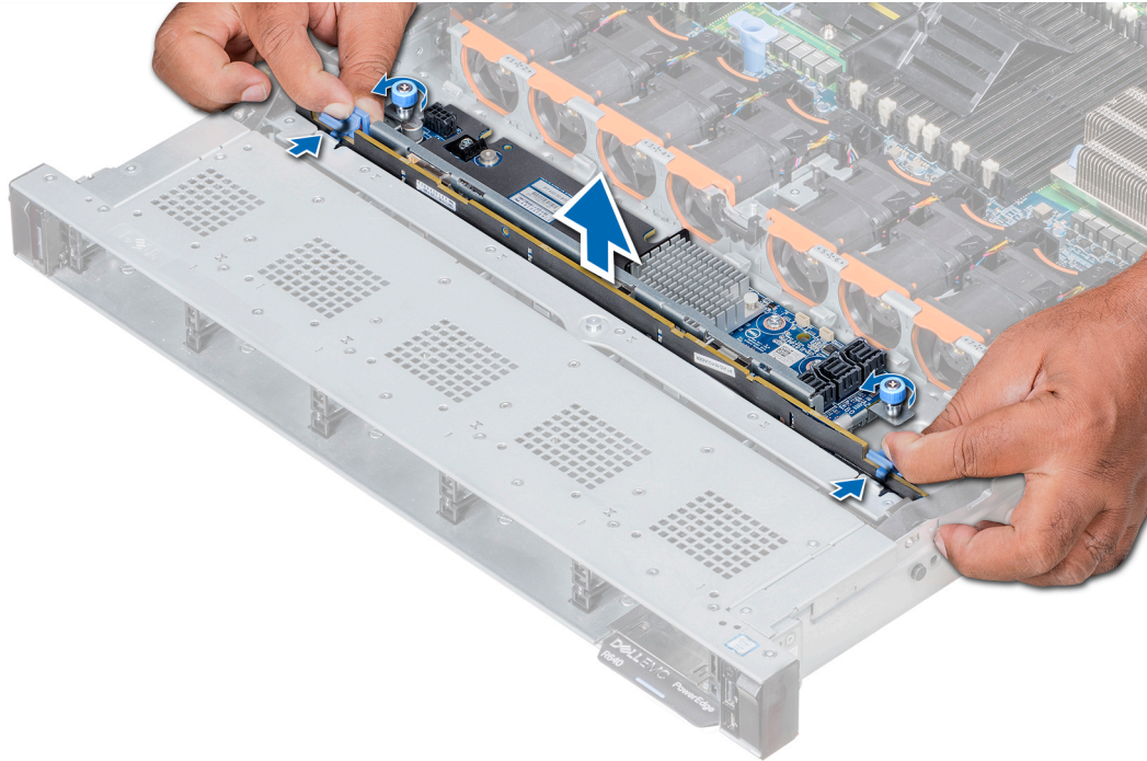
图 59: 卸下硬盘驱动器背板
