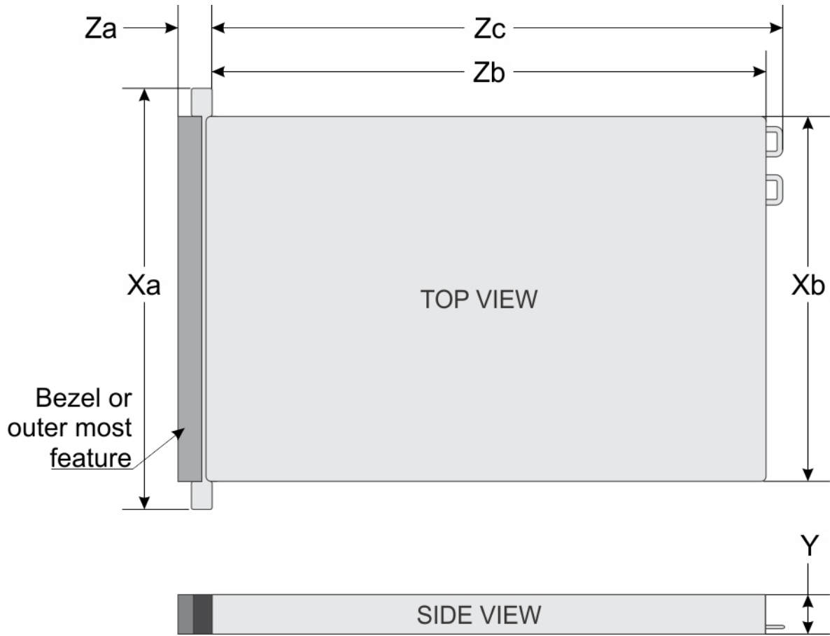
图 13: 系统尺寸
