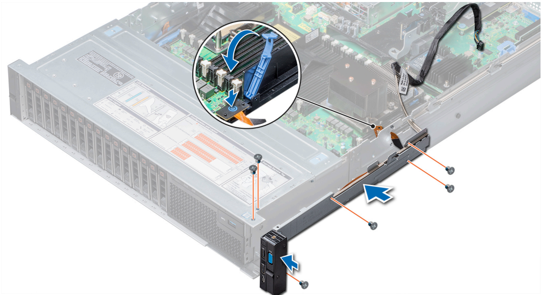
图 82: 安装电缆护套
